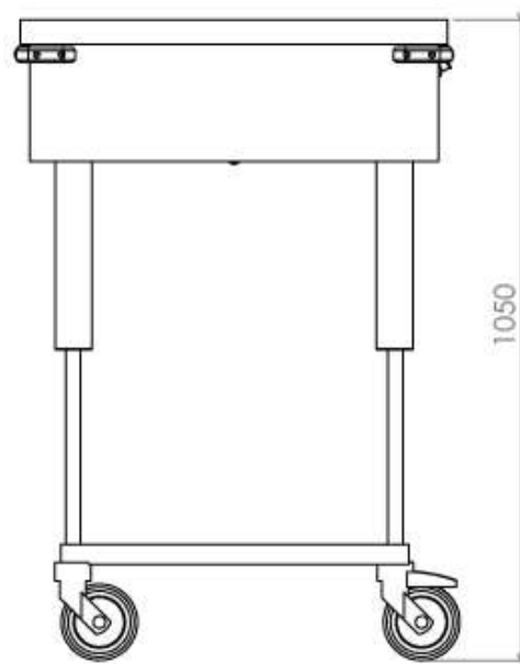
Hauteur Maxi
